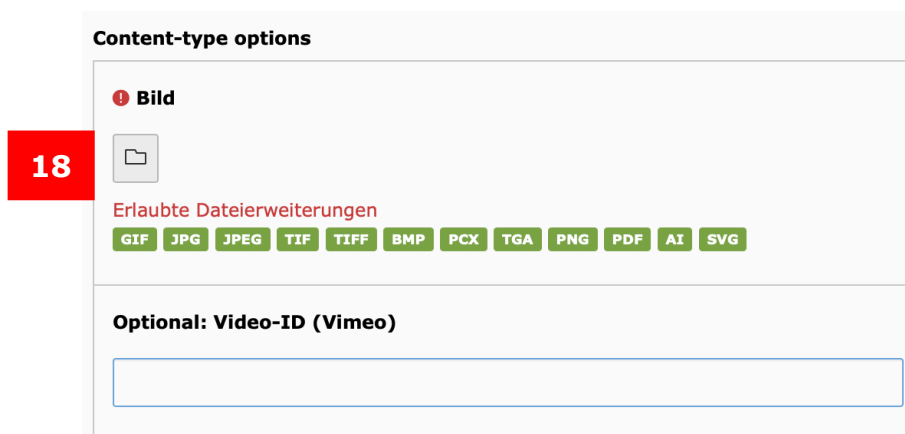
Abbildung 14: Bild hochladen
