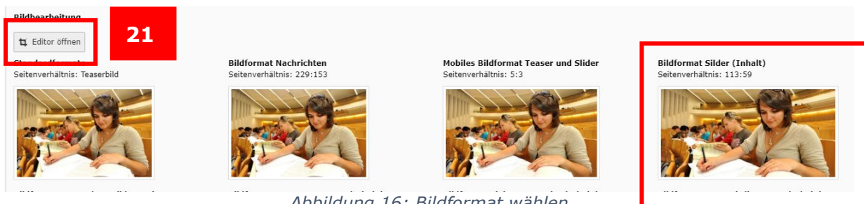
Abbildung 16: Bildformat wählen
