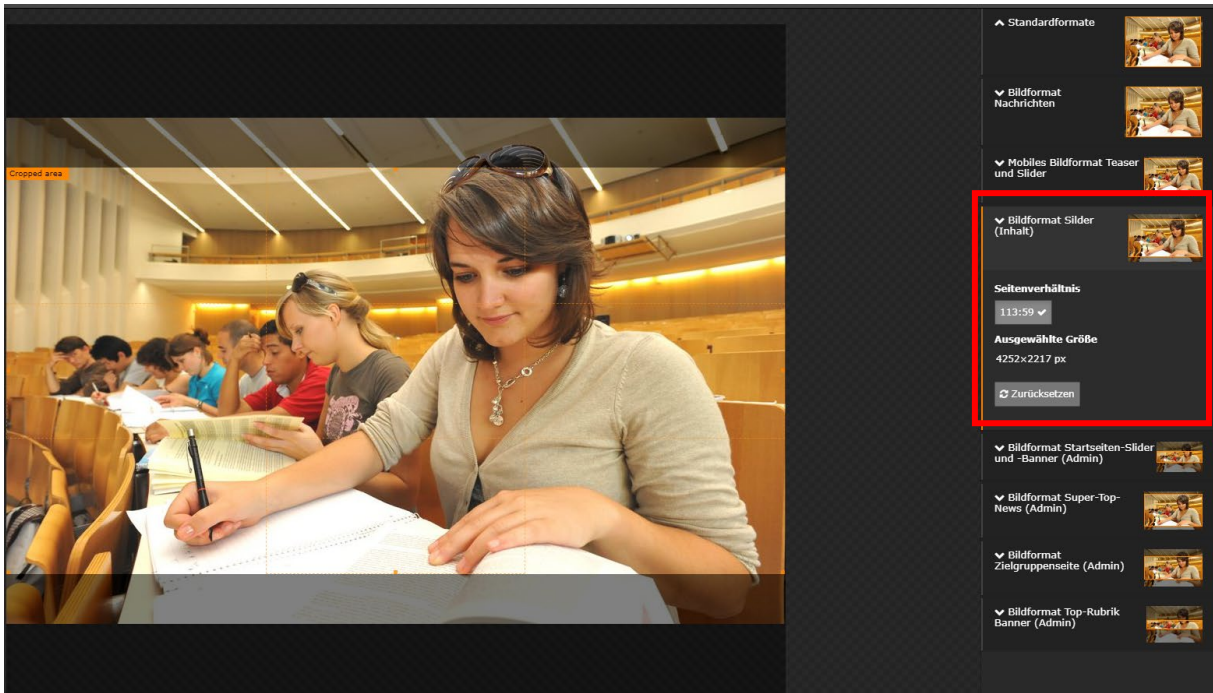
Abbildung 17: Bildausschnitt anpassen
