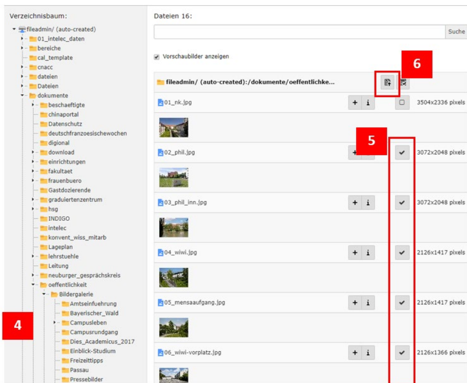
Abbildung 5: Bilder auswählen
