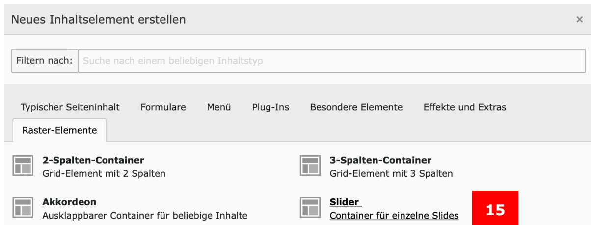
Abbildung 11: Slider-Element anlegen
